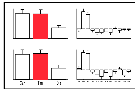
+ Temporal
