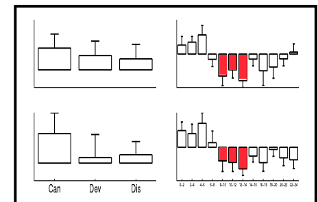
+ FIR
