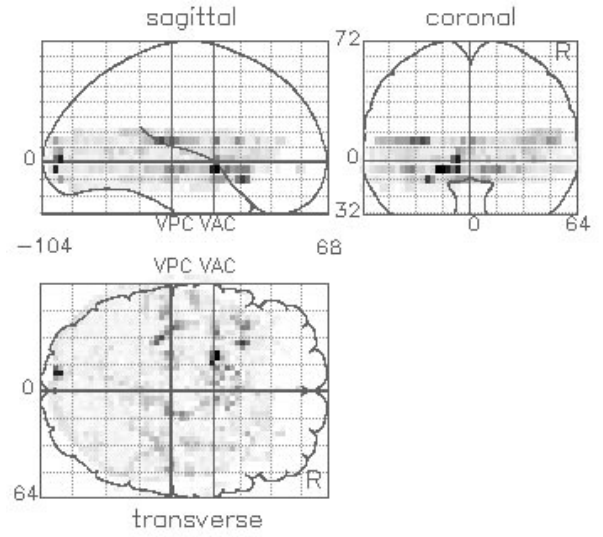
eigenimage 6 {-ve}
