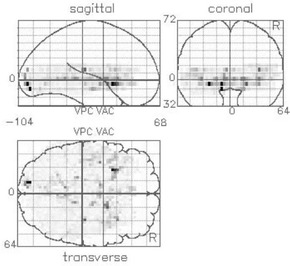
eigenimage 6 {+ve}
